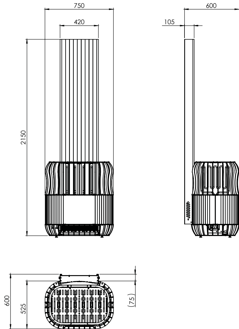
Joonis 1. Saunum Professional mõõdud
